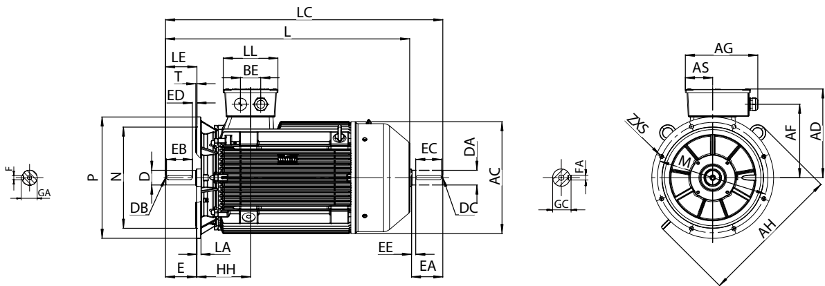
IM B5 以及 IM V1 安装方式 Type of construction IM B5 and IM V1
